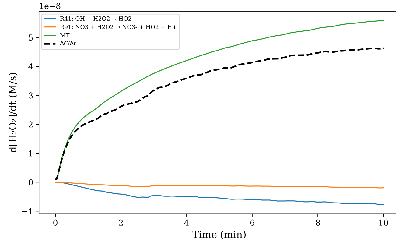
(d) \text{H}_2\text{O}_2
